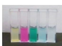
FITC Cy3 Cy5 Cy5.5 Cy7
